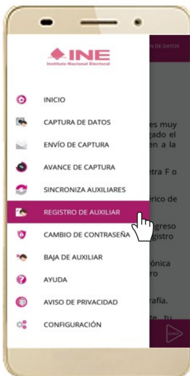
Figura 14. Pantalla de Menú desplegable- Registro de Auxiliar.
